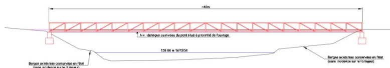
Coupe de principe de la passerelle pour le passage de la piste sur la Zorn
